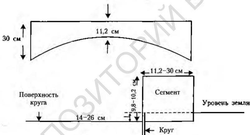
Рис. 19.1. Сегмент для толкания ядра
